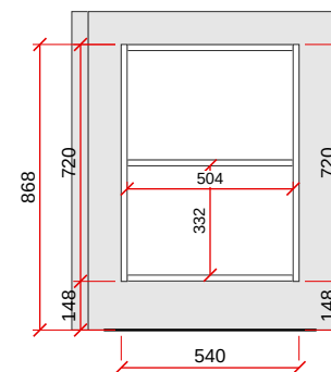
VISTA B - ESC. 1:25
